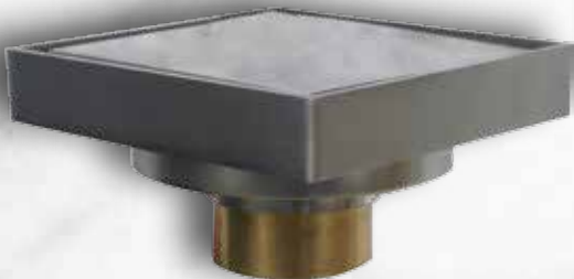
90.5023 A Coladera Cuadrada Acero Inox. 10x10 cm Doble vista (metal/porcelánico).
